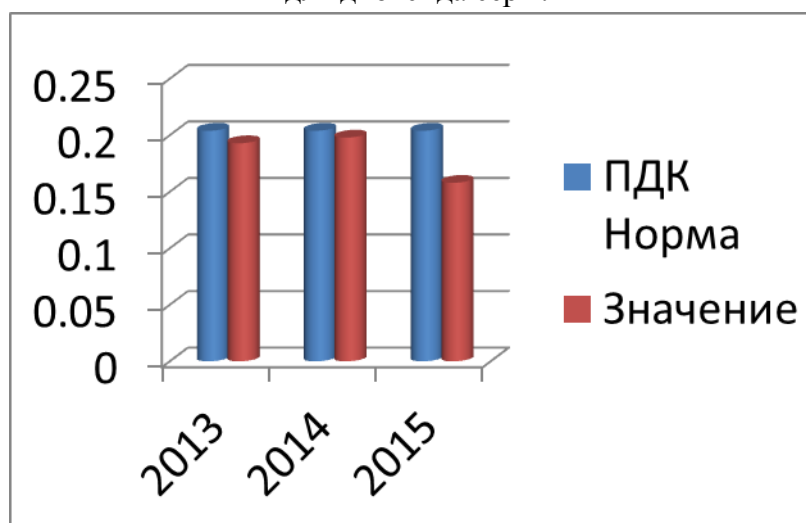
Рис.4. Количество выбросов, производимых предприятием ООО «РРЗ» в динамике для оксида углерода.
