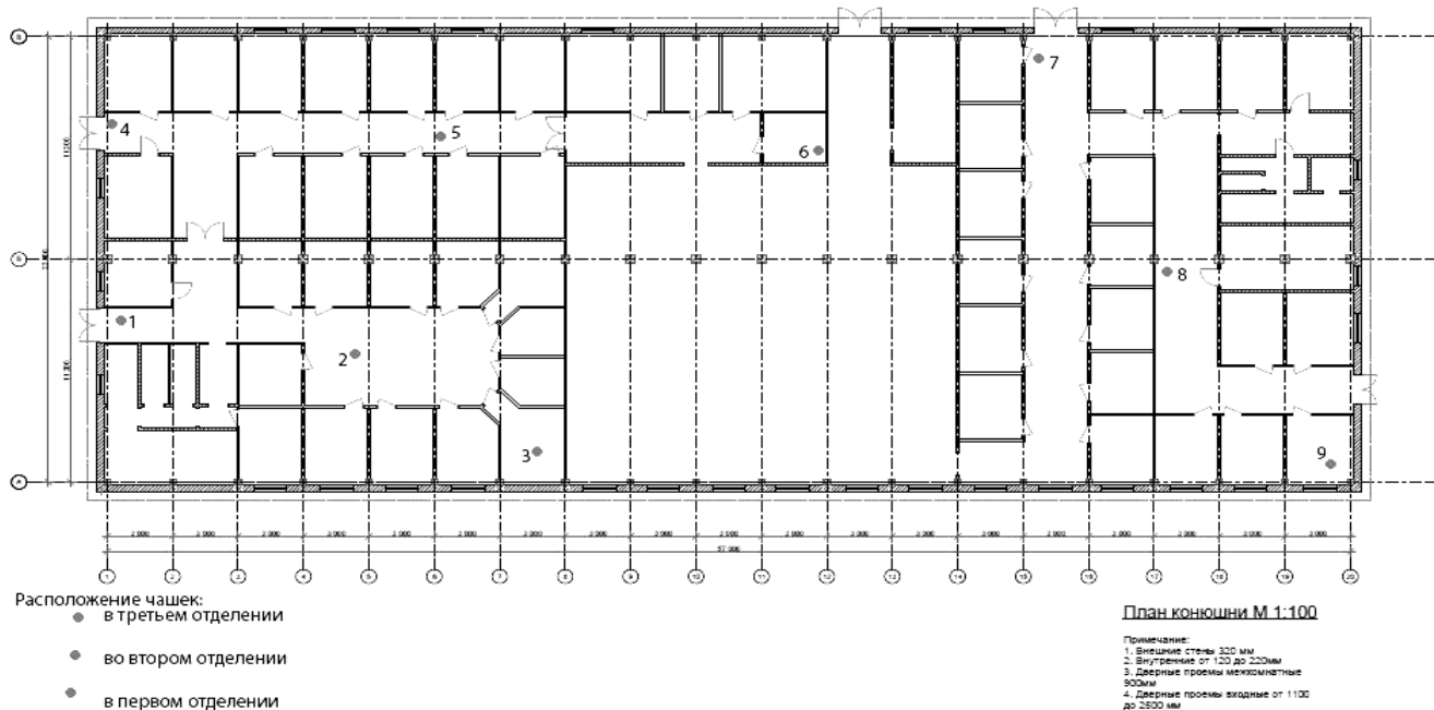
Рис. 1. План КСОЦ «Свобода» с расположением чашек
