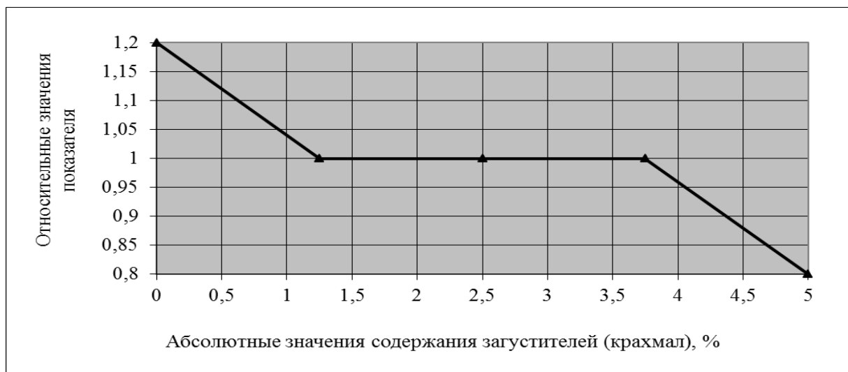
Рис. 6. Содержание загустителей (крахмал). Значение по НД 0,5 %.
