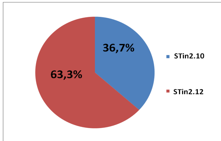
Рис.3. Распределение частот аллелей по полиморфизму STin2 VNTR, локализованного во втором интроне гена транспортера серотонина, у тувинцев.
