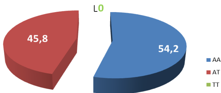
Рис.1. Распределение генотипов по полиморфизму А/Т гена GRO1 у коров голштинской породы, %
