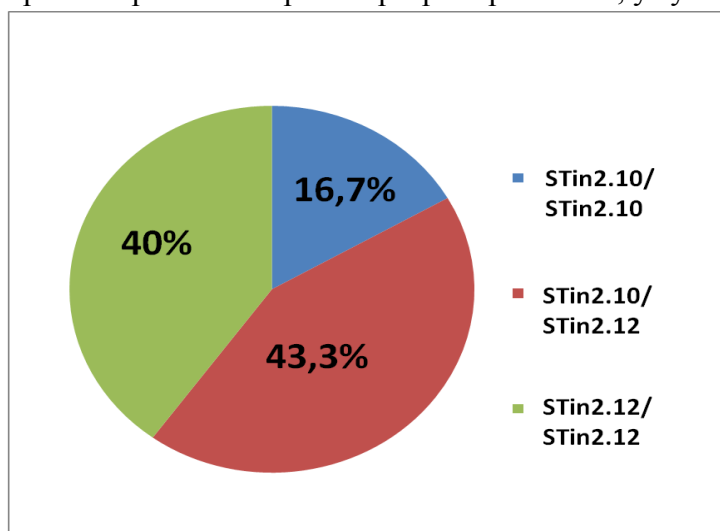
Рис.2. Распределение частот генотипов по полиморфизму STin2 VNTR, локализованного во втором интроне гена транспортера серотонина, у русских.
