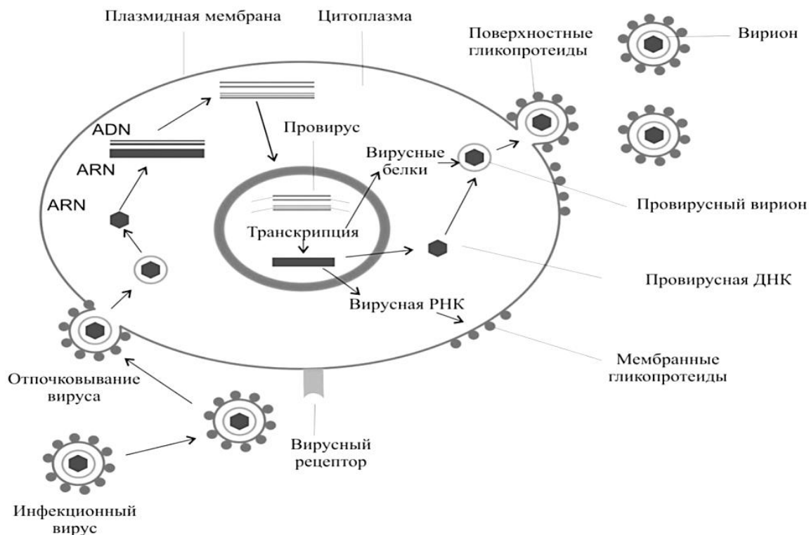
Рис. 1. Схема жизненного цикла репликационно-компетентного ретровируса.
