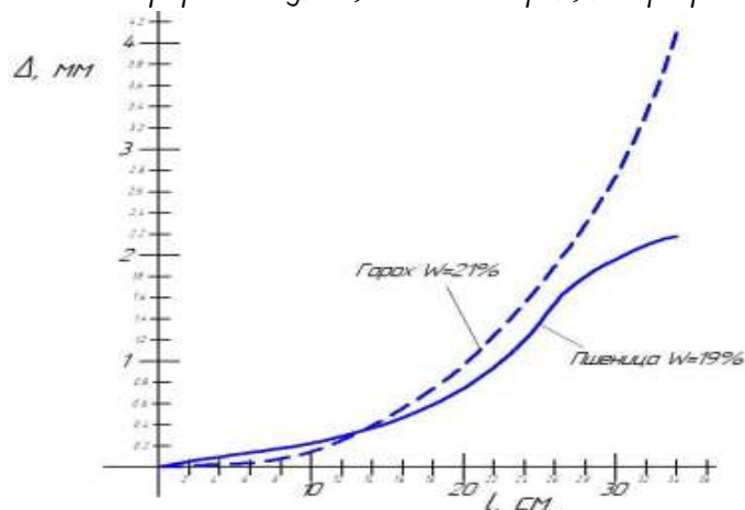
Рисунок 9 - Зависимость величины деформации зерна пшеницы и гороха от длины рабочего пути.
