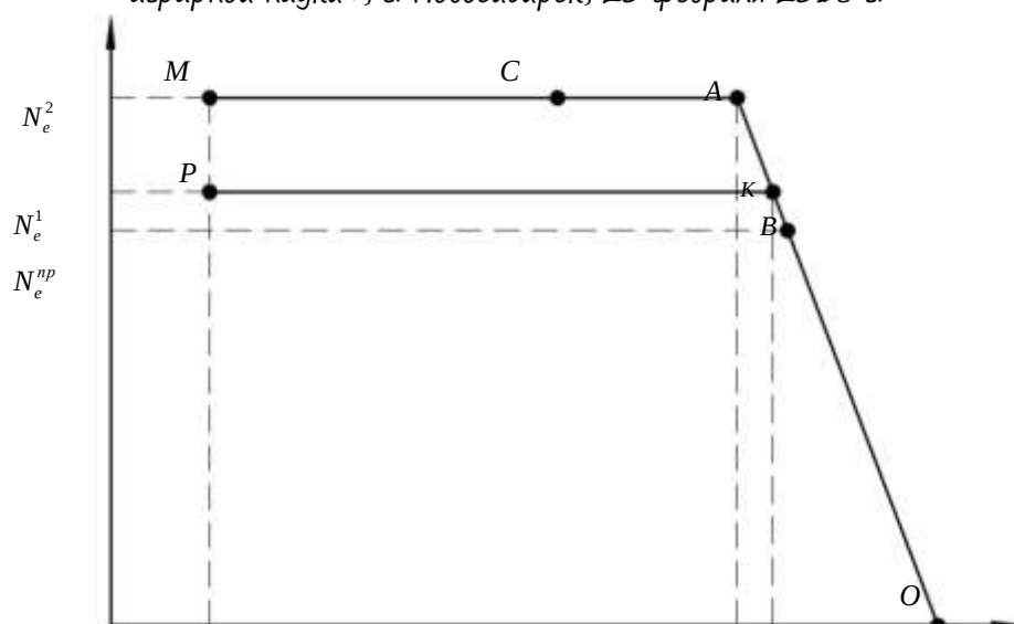
Рисунок 2 – Скоростная характеристика двигателя с двумя уровнями мощности
