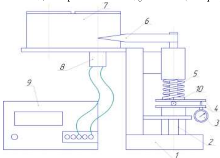
Рис- 1 - Схема прибора для определения величины разрушающего усилия:
