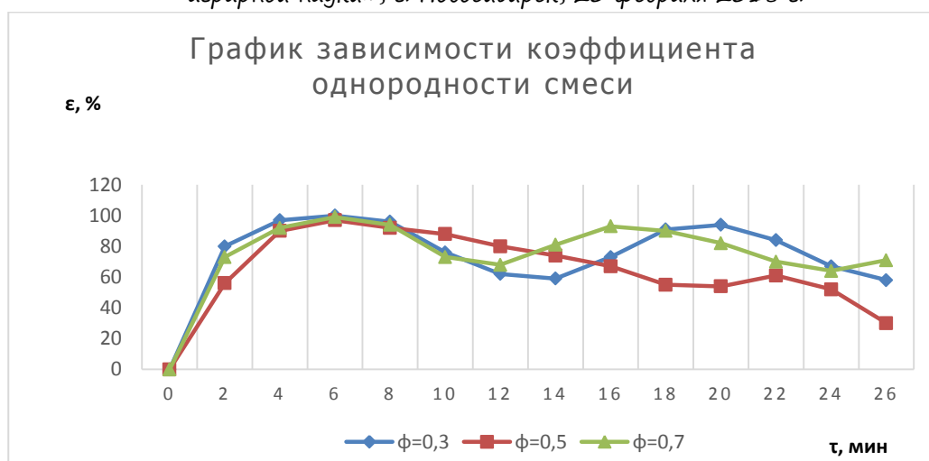
Рисунок 1 – График зависимости коэффициента однородности смеси
