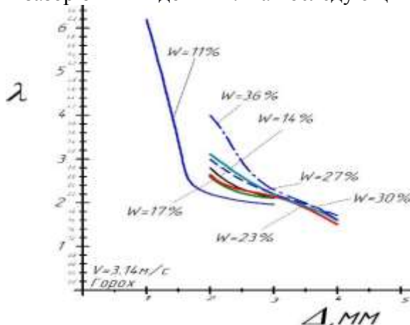
Рисунок 3 - Зависимость степени плющения семян гороха от зазора между вальцами основной зоны.
