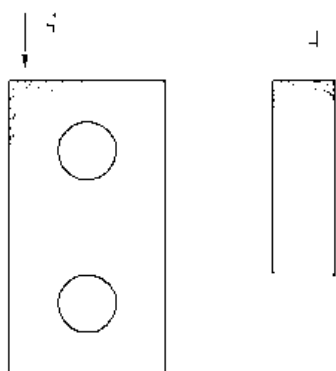
Рисунок 1 – Характер износа молотков
