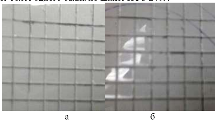
Рисунок 1 – Результаты испытаний адгезионной прочности ремонтного лакокрасочного покрытия
