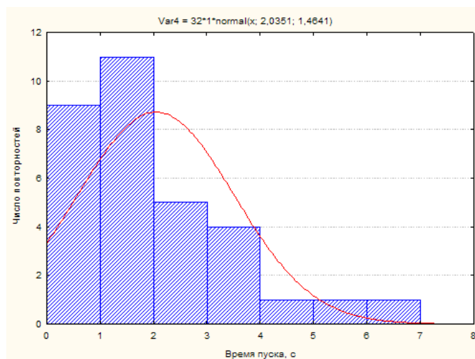
Рисунок 3 – Гистограмма распределения времени пуска прогретого дизеля в условиях эксплуатации
