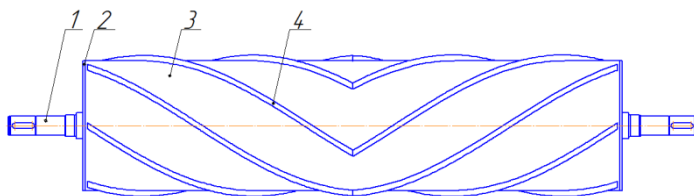
Рисунок 3 – Первый валец прессовальной камеры:
