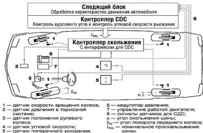
Рисунок 1 – Схема ESP
