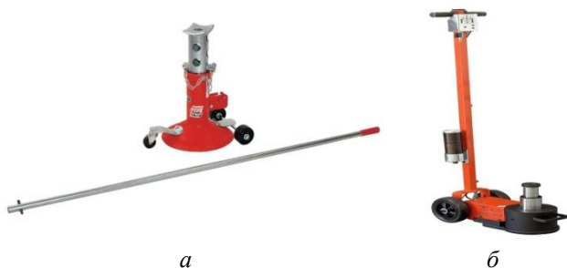
Рисунок 1 – Передвижная опора: а – на роликах; б – на двух колесах
