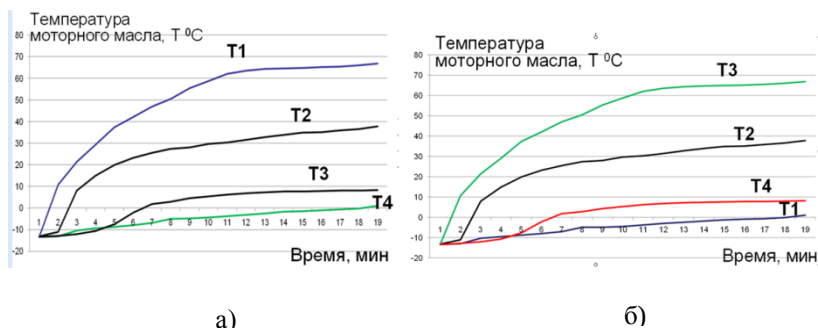
Рисунок 3 – Динамика разогрева моторного масла в картере двигателя СМД-14 электронагревательными устройствами:
