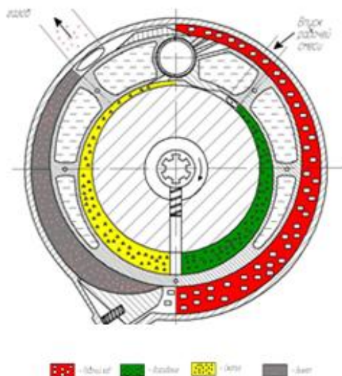
Рисунок 1 – Общая схема работы роторного двигателя РДТ (первый вариант)
