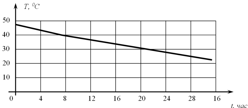
Рисунок 5 - График остывания моторного масла в гидроаккумуляторе (температура окружающей среды T=-18 \dots -23 °C)
