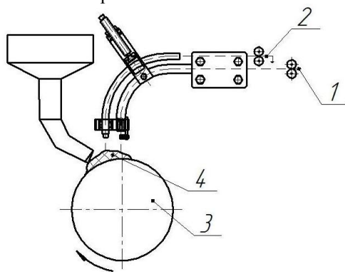
Рисунок 1 – Схема наплавки двумя проволоками: 1 – основная проволока; 2 – присадочная проволока; 3 – деталь; 4 – флюс
