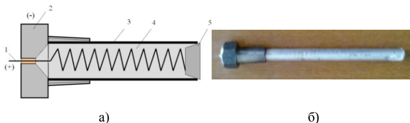
Рисунок 1 - Устройство для разогрева моторного масла: а – схема устройства; б – внешний вид устройства; 1 – спираль; 2 – штуцер; 3 – корпус; 4 – кварцевый песок; 5 – пробка
