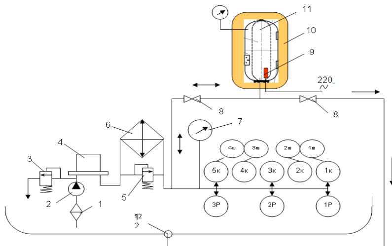
Рисунок 1 – Схема устройства для предпусковой подачи масла в систему смазки двигателя Д-240:
