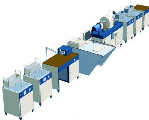
Рисунок 1 – Участок входного контроля подшипников качения
