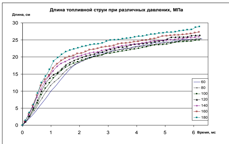
Рисунок 2 - Экспериментальные значения длины топливной струи при различных давлениях впрыска для дизельного топлива.
