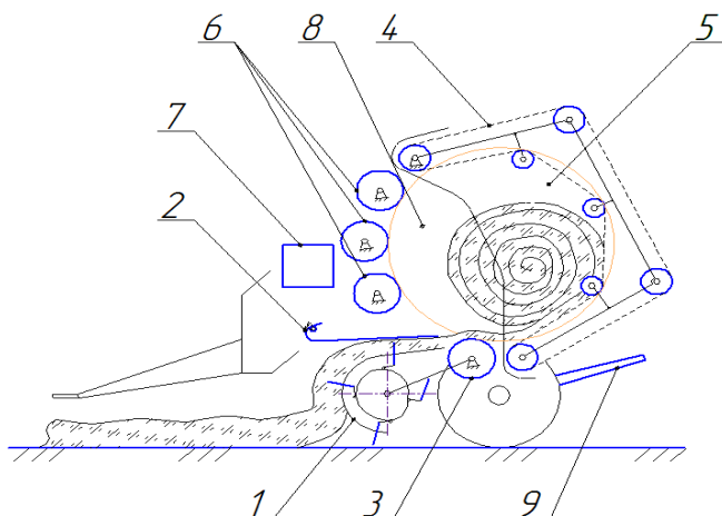
Рисунок 2 – Схема усовершенствованного пресс-подборщика для применения цепочного транспортера без роликов на планках:
