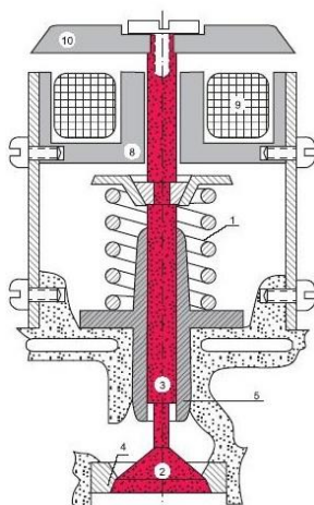
Рисунок 2 - Схема электромагнитного клапана с возвратной пружиной:
