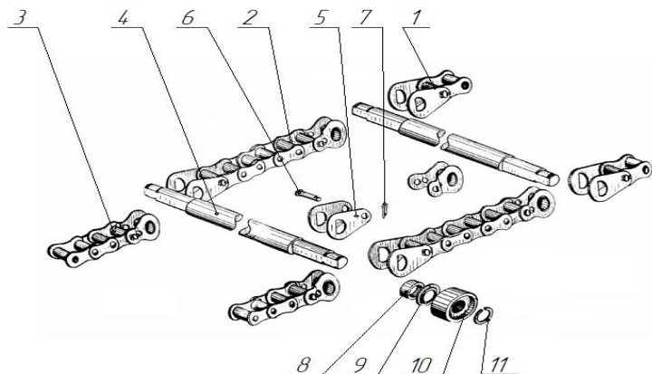
Рисунок 5 – Устройство замкнутого цепочно-пруткового транспортера:
