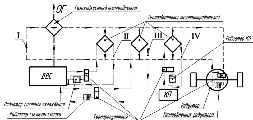
Рисунок 2 – Функциональная схема системы автоматического поддержания оптимальных температур рабочих жидкостей и масел в основных агрегатах и узлах самоходных машин: I – контур утилизационный; II – контур теплопотребления системы охлаждения ДВС; III – контур теплопотребления системы смазки ДВС; IV – контур теплопотребления системы смазки КП
