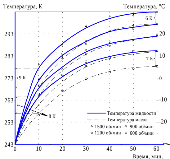
Рисунок 2 – Динамика температуры промежуточного теплоносителя и трансмиссионного масла при различной частоте вращения коленчатого вала
