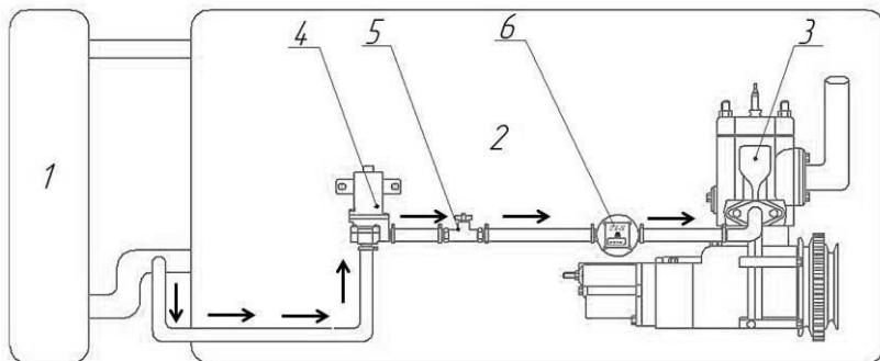
Рисунок 2 – Схема циркуляции жидкости в подогреваемой магистрали: 1 – радиатор; 2 – ДВС (СМД-14); 3 – пусковой двигатель (ПД-10); 4 – жидкостный насос (12В); 5 – вентиль; 6 – расходомер жидкости
