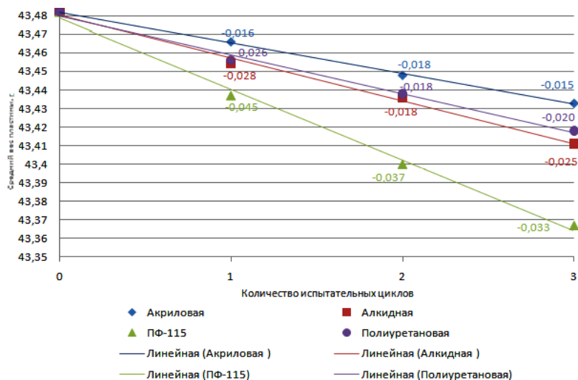
Рисунок 4. – Истираемость лакокрасочных покрытий (эмаль + эпоксидный грунт)
