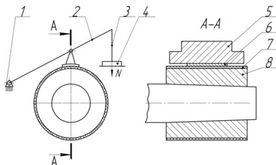
Рисунок 1 – Схема нагрузочного узла машины трения УРБ-ВП
