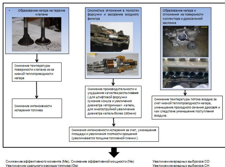
Рисунок 1 – Влияние отложений на выходные параметры ДВС
