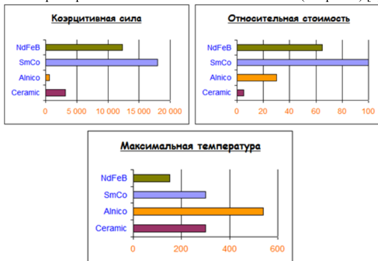
Рисунок 4- Характеристики классов магнитов по показателям [4,5,6]
