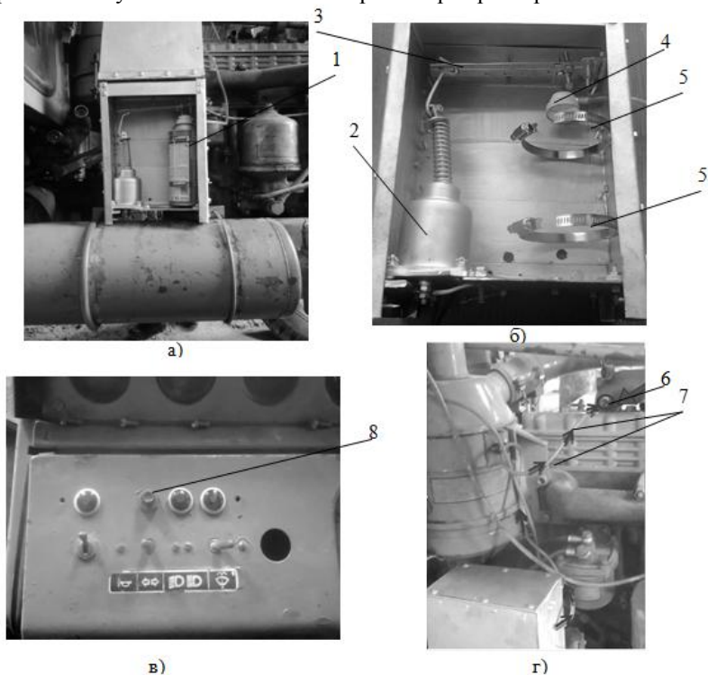
Рисунок 2 - Устройства для подачи легковоспламеняющейся жидкости из аэрозольного баллона во впускной коллектор:
