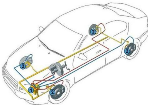
Рисунок 1 - Устройство ABS
