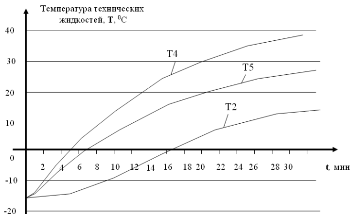
Рисунок 3 – Динамика разогрева технических жидкостей двигателя СМД-14 электрическим подогревателем (скорость потока жидкости через теплообменник S=5 л/мин; мощность нагревательного элемента N=3 кВт; температура окружающей среды T=-17^{\circ}\text{C} )
