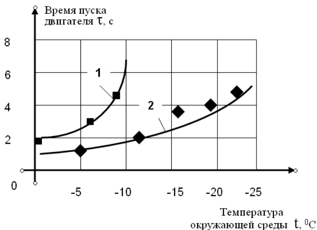
Рисунок 3 – Зависимость времени пуска двигателя Д-240 от температуры окружающей среды:
