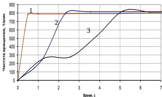
Рисунок 1 - Динамика пуска дизеля D4EB автомобиля Hyundai SantaFe с системой Common Rail:
