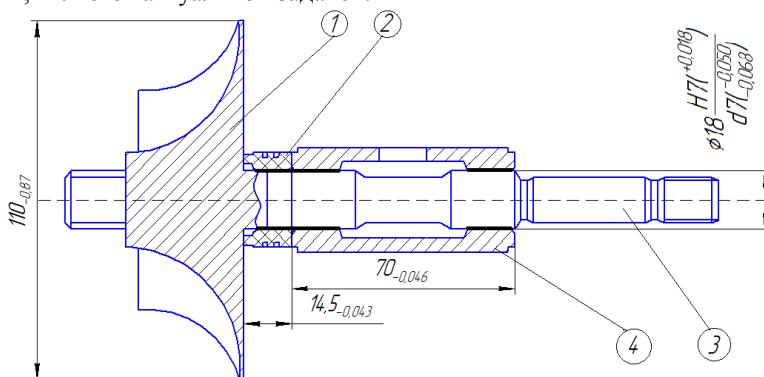
Рисунок – Соединение вал ротора – подшипник:
