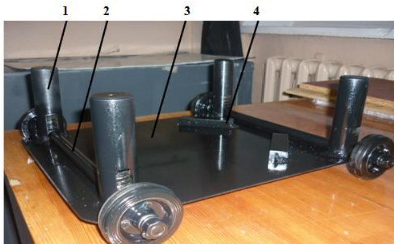
Рисунок 2 – Передвижная опора с пружинной подвеской: 1 – стакан с упругим элементом; 2 – ось; 3 – платформа; 4 – прилив
