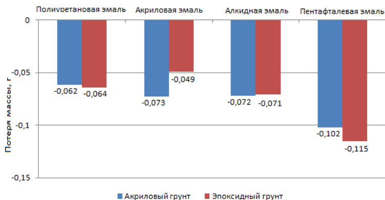
Рисунок 5 – Истираемость различных систем лакокрасочных покрытий.
