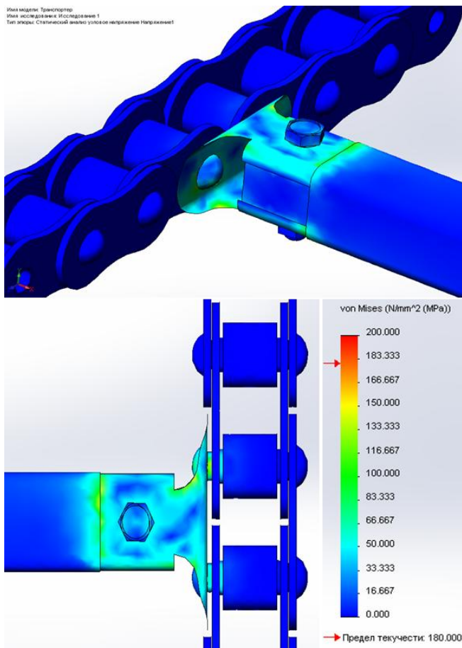
Рисунок 4 - Распределение напряжений
