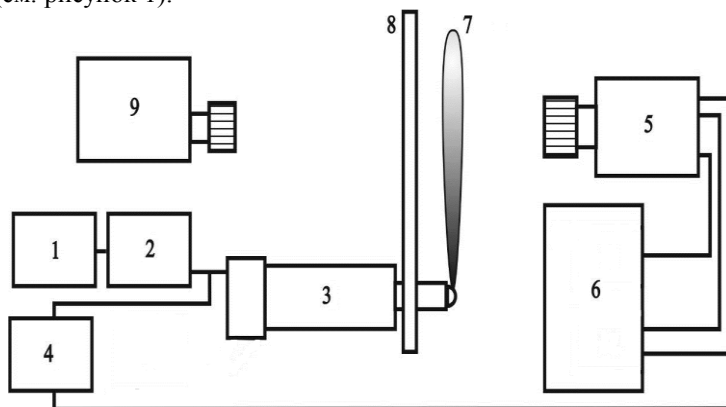
Рисунок 1 - Схема стенда скоростной видеосъемки.
