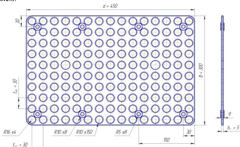
Рисунок 2 - Пластина-носитель диоксида титана
