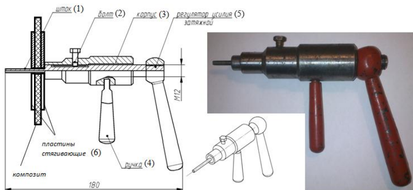
Рисунок 1 - Приспособление для фиксации ремонтируемого участка
