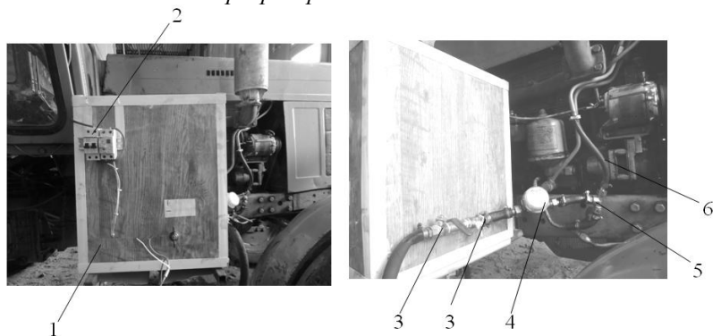
Рисунок 2 - Устройство для предпусковой подачи масла в систему смазки двигателя Д-240:
