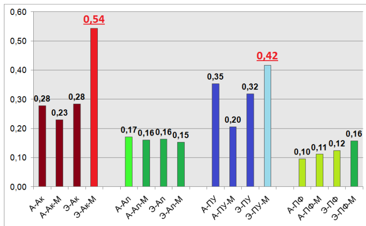
Рисунок 2 - Адгезионная прочность различных вариантов эмалей, МПа
