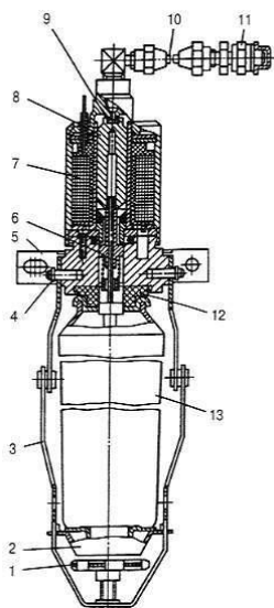
Рисунок 1 – Аэрозольное пусковое приспособление с электромагнитным приводом: 1 – регулировочный винт; нажимной подпятник; 3 – складывающиеся душки; 4 – ось душек; 5 – кронштейн крепления; 6 – эмульсионная трубка; 7 – электромагнит; 8 – сердечник; 9 – пластинчатый клапан; 10 – коллектор; 11 – форсунка; 12 – резиновый уплотнитель; 13 – аэрозольный баллон
