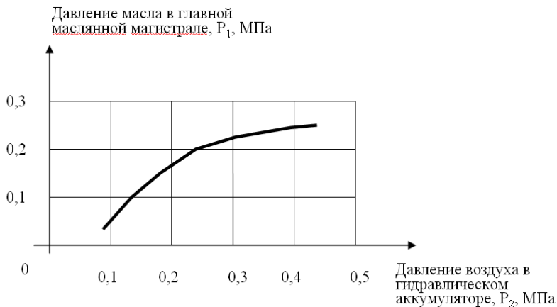
Рисунок 3 – Зависимость давления в главной масляной магистрали от давления воздуха в гидравлическом аккумуляторе (температура моторного масла в гидравлическом аккумуляторе 38 - 42^{\circ}\text{C} , температура окружающей среды -18 \dots -24^{\circ}\text{C} , марка моторного масла М-10Г 2 )
