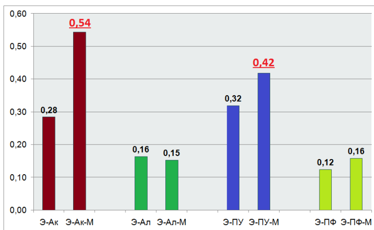
Рисунок 4 - Адгезионная прочность эмалей на эпоксидном грунте, МПа
