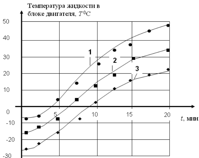
Рисунок 2 – Интенсивность разогрева охлаждающей жидкости в блоке двигателя СМД-14 предпусковым бензиновым подогревателем (подача насоса S=5 л/мин):
