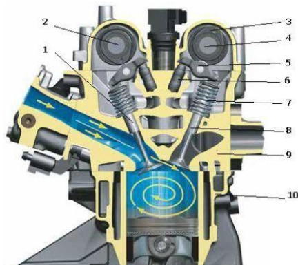
Рисунок 1 - Схема ГРМ четырехтактного двигателя:
