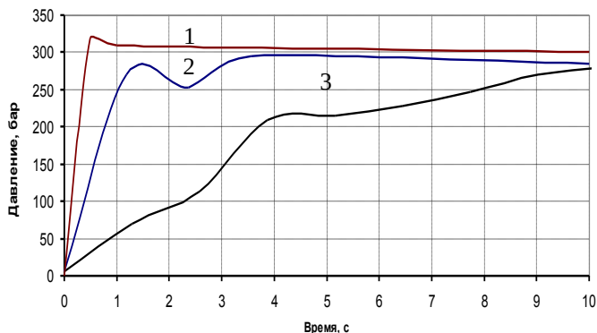
Рисунок 2 - Динамика набора давления в аккумуляторе системы Common Rail дизеля D4EB автомобиля Hyundai SantaFe:
