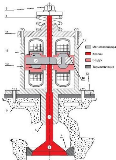
Рисунок 3 - Схема электромагнитного клапана без возвратной пружины: 1 - пружина; 2 - клапанная головка; 3 - клапанный стержень; 4 - посадочная фаска; 5 - направляющая втулка; 6 - электромагнит открывающий; 7 - якорь; 8 - электромагнит закрывающий; 9 - натяжная гайка; 10 - зажимные трубки; 11 - немагнитная крышка; 12 - гильза; 13 - термоизоляционная прокладка; 14 - головка блока цилиндров
