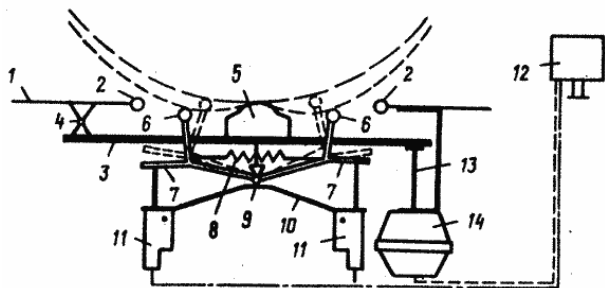
Рисунок 3 - Схема работы стенда:
