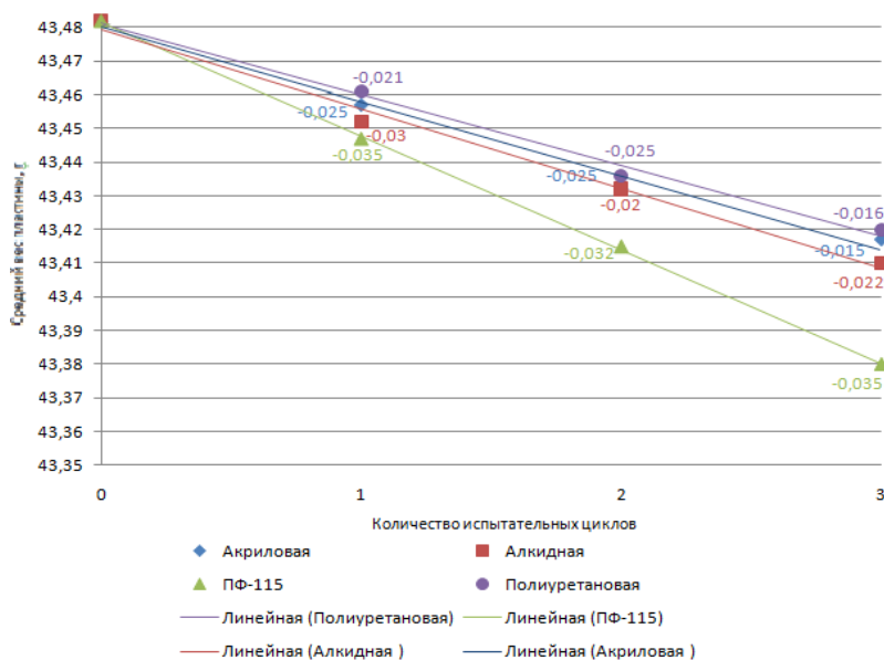
Рисунок 3 – Истираемость лакокрасочных покрытий (эмаль + акриловый грунт)
