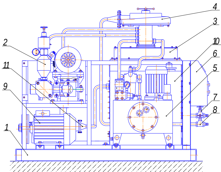
Рисунок 1 – Общий вид экспериментального стенда для центробежной очистки гидравлических масел оборудованный: 1 – рама; 2 – компрессор; 3 – привод центробежного очистительного устройства; 4 – исследуемое центробежное очистительное устройство; 5 – насосная станция; 6 – пульт управления; 7 – заборный вентиль; 8 – отводной вентиль; 9 – электродвигатель; 10 – масляный нагреватель; 11 – центробежный насос.
