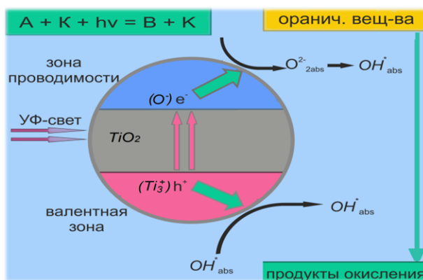
Рисунок 3 – Принцип фото-катализа
