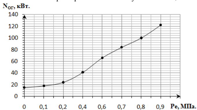
Рисунок 1 – Зависимость мощности теплового потока отработанных газов от степени загрузки двигателя
