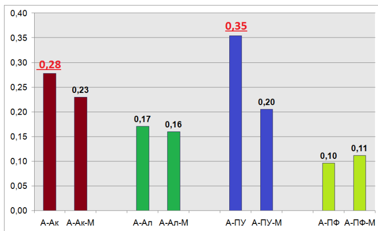
Рисунок 3 - Адгезионная прочность эмалей на акриловом грунте, МПа
