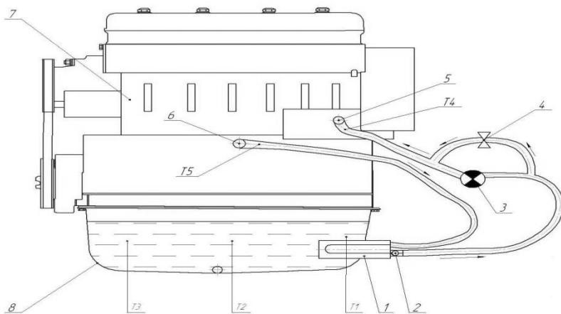
Рисунок 2 – Схема установки электрического предпускового подогревателя в масляный картер двигателя СМД-14:
