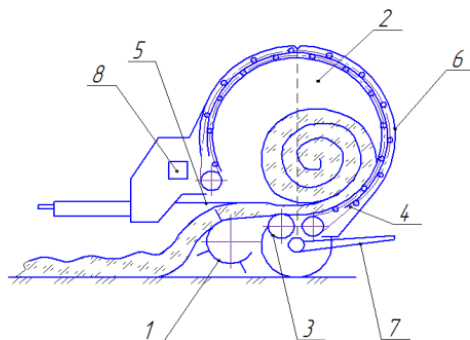
Рисунок 1 – Технологическая схема пресс-подборщика ПР-Ф-145 1 - подборщик; 2 - прессовальная камера; 3 - барабан; 4 - цепочно-планчатый транспортер; 5 - прижимная решетка; 6 - задняя часть камеры прессования; 7 - рамка; 8 - вязальный аппарат
