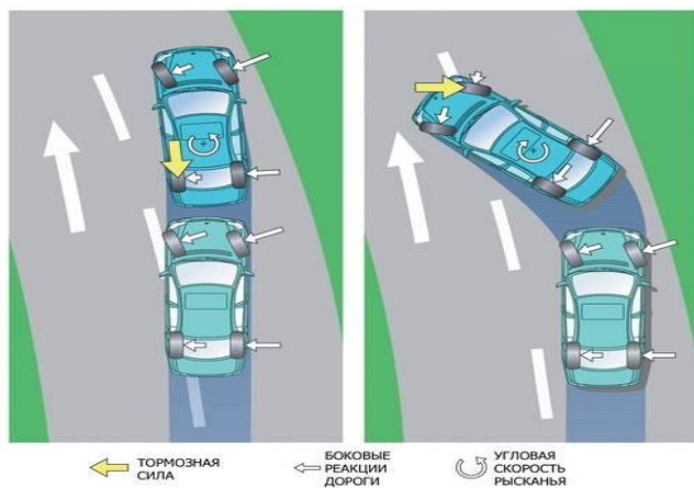
Рисунок 2 – Траектория автомобиля с ESP и без нее
