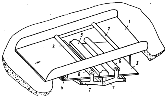
Рисунок 2 – Стенд для измерения давления в пневматических шинах транспортного средства:
