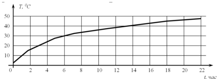
Рисунок 4 - График нагрева моторного масла в гидравлическом аккумуляторе (мощность нагревательного устройства N=30 Вт, температура окружающей среды T=-20 \dots -25 °C)
