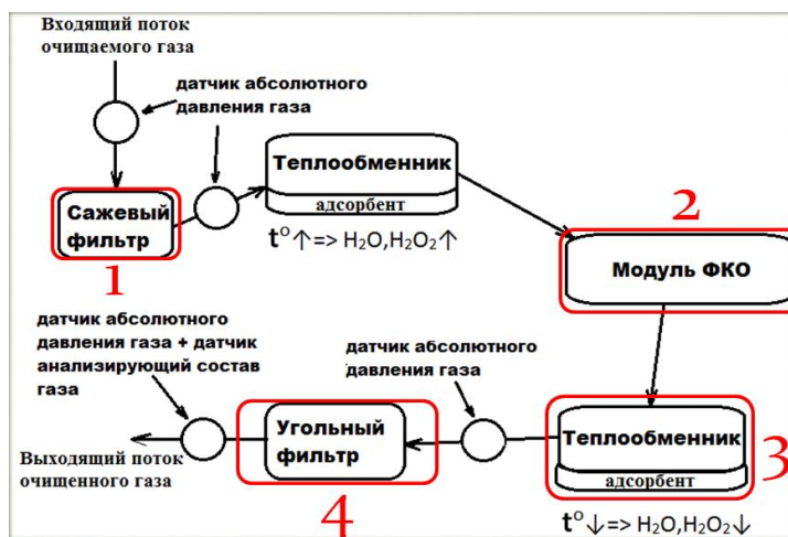
Рисунок 5 – Блок-схема устройства
