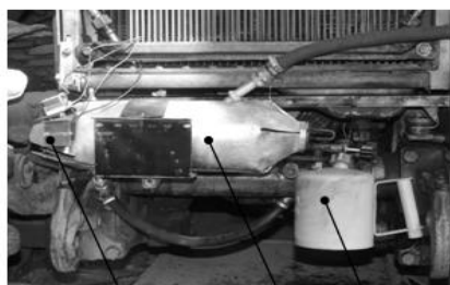
Рисунок 1 – Предпусковой подогреватель ДВС на базе бензиновой горелки: а – схема устройства; б – установка предпускового подогревателя на трактор ДТ-75НБ; 1 – спирально-трубчатый подогреватель; 2 – бензиновая горелка; 3 – термоэлектрический генератор (элемент Пельтье)
