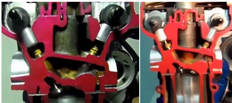
Рисунок 5 - Компоновка двигателя (система DOHC) с применением постоянных магнитов
