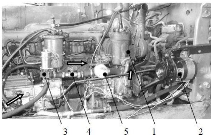
Рисунок 1 – Предпусковой разогрев охлаждающей жидкости двигателя СМД-14 путем утилизации тепла от пускового устройства ПД-10:
