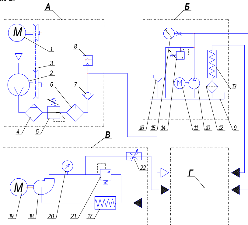
Рисунок 2 – Принципиальная гидравлическая схема экспериментального стенда: (А – пневматическая система) 1 – электромотор компрессора; 2 – компрессор; 3 – клиноременная передача; 4 – фильтр влагоотделитель; 5 – редукционный клапан; 6 – масляный распылитель; 7 – клапан; 8 – реле давления; (Б – привод системы смазки) 9 – бак; 10 – насос пластинчатый; 11 – клапан; 12 – клапан; 13 – клапан; 14 – датчик; 15 – манометр; 16 – трубопровод; (В – гидродинамический привод) 17 – трубопровод; 18 – насос; 19 – электромотор; 20 – манометр; 21 – клапан; 22 – редукционный клапан.
