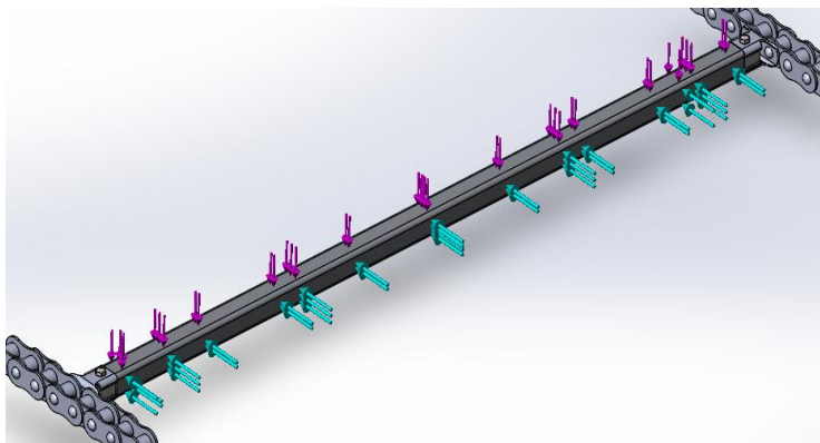
Рисунок 2 – Схема сил, действующих на планку:
