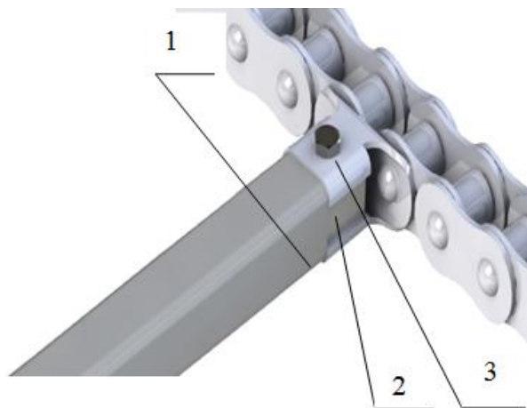
Рисунок 1 – 3D – модель модернизированного цепочно-планчатого транспортера:
