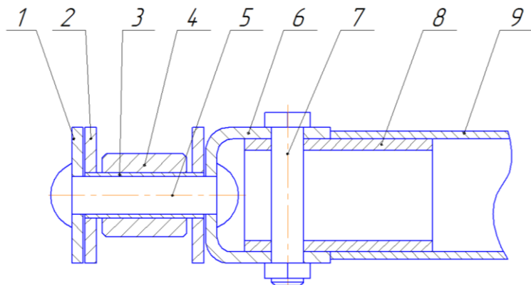
Рисунок 6 – Схема предлагаемой модернизированной конструкции: 1 – наружная пластина; 2 – внутренняя пластина; 3 – втулка; 4 – ролик; 5 – заклепка; 6 – соединительная пластина; 7 – болтовое соединение; 8 – удлинитель; 9 – планка
