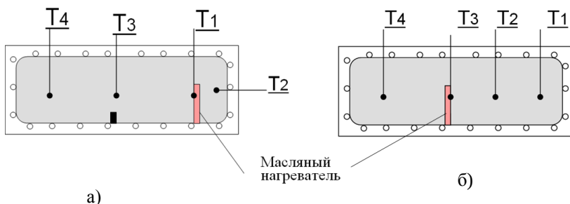
Рисунок 3 – Схема установки температурных датчиков в масляном картере двигателя СМД-14:
