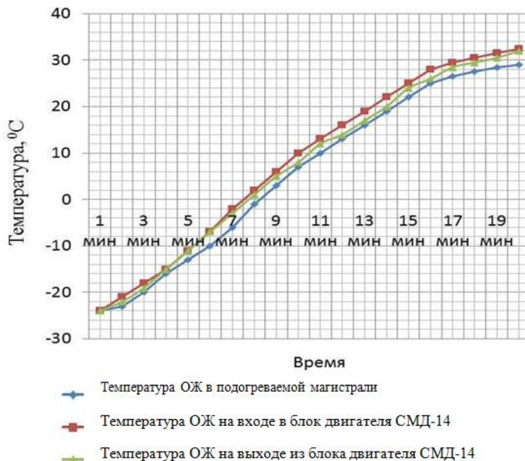
Рисунок 3 – Динамика предпускового разогрева охлаждающей жидкости двигателя СМД-14 (при температуре окружающей среды t = -24^{\circ}\text{C} , подача насоса S=5 л/мин.)
