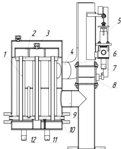
Рисунок 3 – Рекуперативный кожухотрубный газожидкостный теплообменник с автоматической системой управления процессом теплообмена (обозначение позиций см. по тексту)
