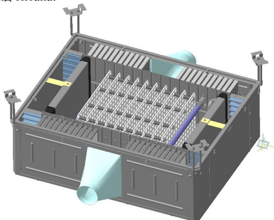
Рисунок 1 – Устройство очистки газов (без верхней крышки)
