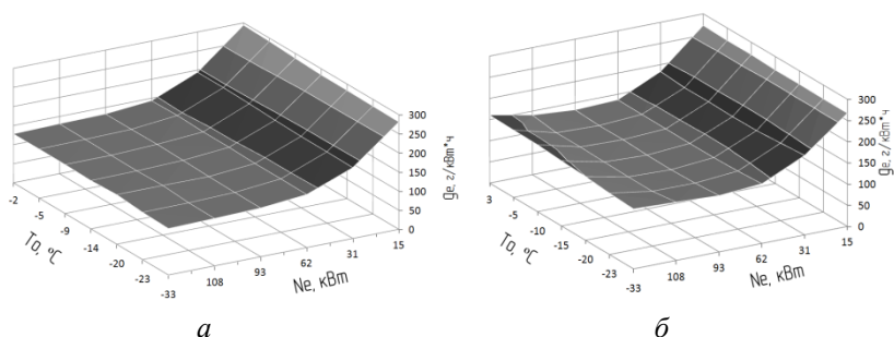
Рисунок 2 – Зависимость удельного эффективного расхода топлива от температуры окружающей среды и загрузки двигателя по мощности N_e : а – с включённым наддувом; б – без наддува.
