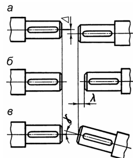
Рис. 2.20. Погрешности монтажа валов:
