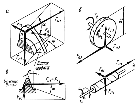
Рис. 3.13. Схема сил, действующих в червячном зацеплении
