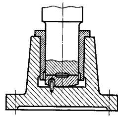
Рис. 2.11. Подпятник
