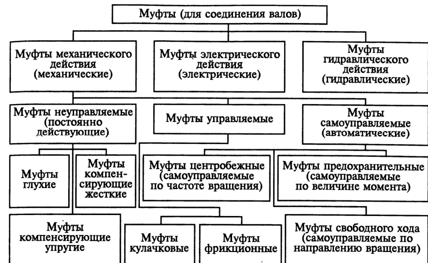
Рис. 2.17. Классификация муфт
