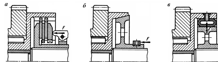
Рис. 2.26. Схемы фрикционных муфт
