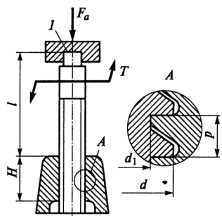
Рис. 3.29 — Схема нагружения винта домкрата
