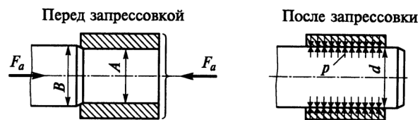
Рис.1.37 - Расчетная схема соединения с натягом
