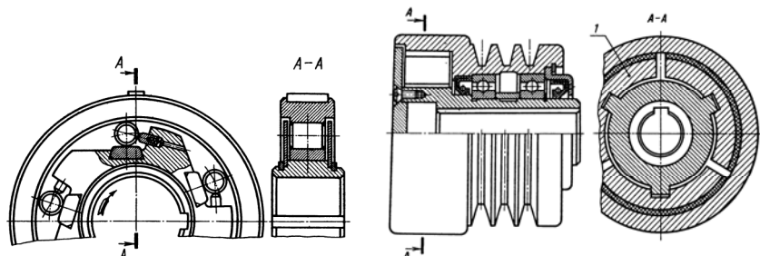
Рис. 2.27. Муфта обгонная
