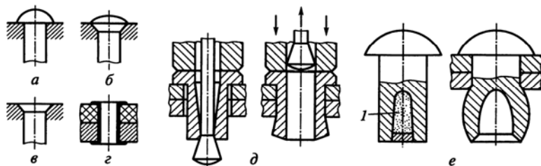
Рис. 1.18. Типы заклепок
