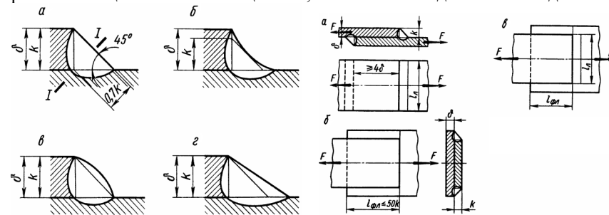
Рис. 1.22. Угловые швы
