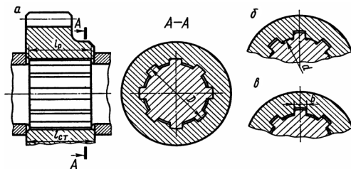
Рис. 1.30. Шлицевое соединение
