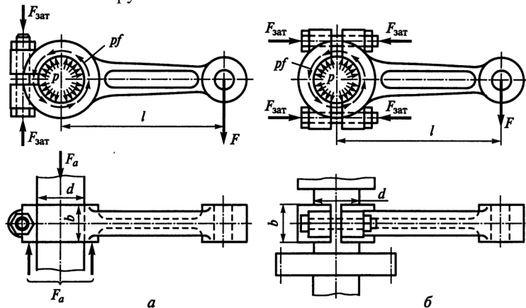
Рис 1.42 - Клеммовые соединения
