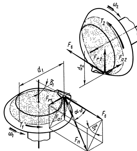
Рис. 3.8. Схема сил в конической прямозубой передаче (колеса условно раздвинуты)
