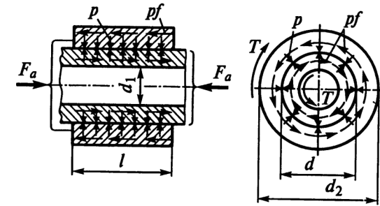
Рис. 1.38 – К расчету соединения с натягом
