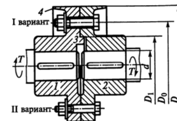
Рис. 2.19. Фланцевая муфта
