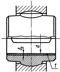
Рис. 2.10. Самоустанавливающийся подшипник: 1 – баббитовая заливка
