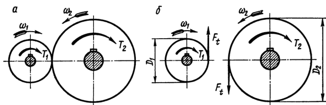
Рис. 3.1. Схема для определения направления вращающих моментов в передаче: а – колеса в рабочем положении; б – колеса, условно раздвинутые
