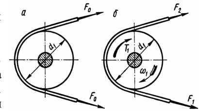
Рис. 3.16. Силы в ветвях ремня
