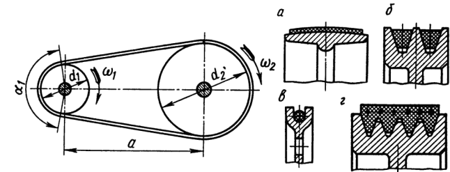
Рис. 3.14. Схема ременной передачи
