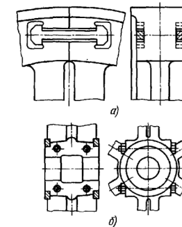
Рис. 1.36. Соединение половин маховиков по плоскости
