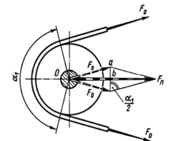
Рис. 3.17. К определению нагрузки на валы ременной передачи
