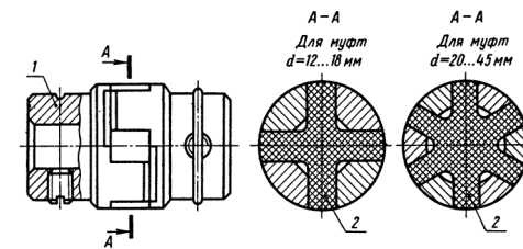
Рис. 2.24. Муфта упругая со звездочками
