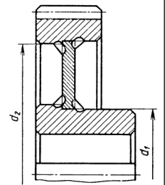
Рис. 1.25. Сварное зубчатое колесо
