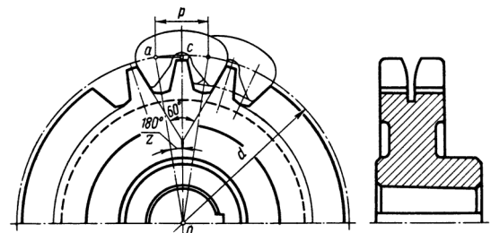
Рис. 3.24. Звездочка зубчатой цепи
