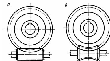
Рис. 3.10. Схемы червячных передач
