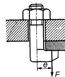
Рис. 1.16. Эксцентричная нагрузка
