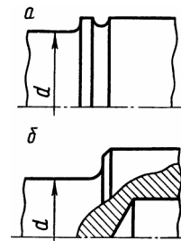
Рис. 2.6. Способы повышения усталостной прочности валов
