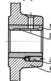
Рис. 2.8. Неразъемный подшипник: 1 – втулка; 2 – смазочная канавка; 3 – стопорный винт; 4 – станина
