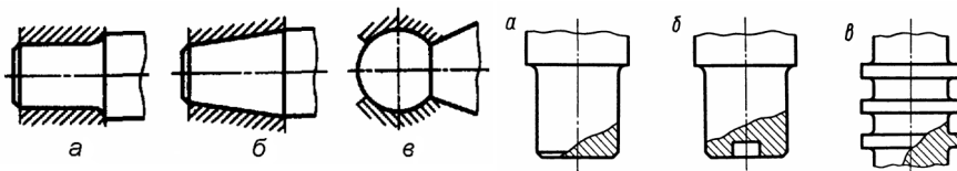
Рис. 2.3. Основные типы цапф под подшипники скольжения
