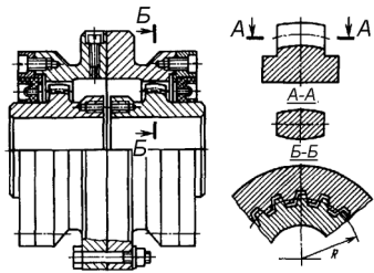
Рис. 2.21. Зубчатая муфта
