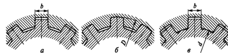
Рис. 1.32. Способы центрирования
