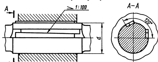
Рис. 1.29. Соединения тангенциальными шпонками
