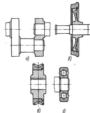
Рис. 1.35. Соединение с натягом по цилиндрическим поверхностям
