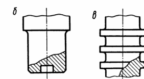
Рис. 2.4. Пяты
