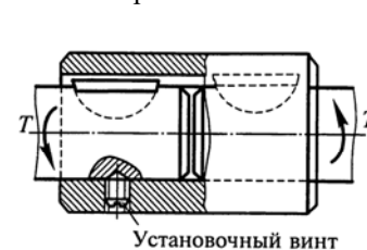
Рис. 2.18. Втулочная муфта
