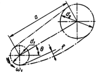
Рис. 3.25. Схема цепной передачи
