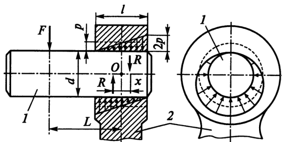
Рис. 1.39 - Эпюра давлений в соединении при нагружении изгибающим моментом
