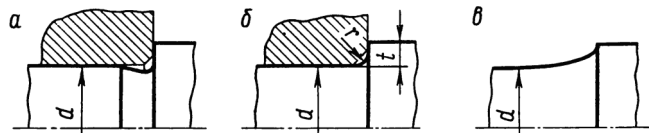
Рис. 2.5. Переходные участки вала
