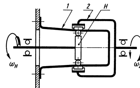
Рис. 3.31 – Схема волновой передачи движения в герметизированном пространстве
