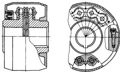
Рис. 2.22. Цепная муфта
