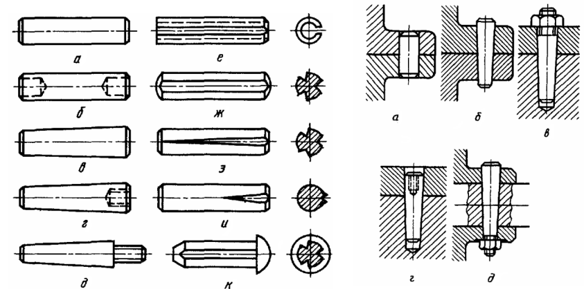
Рис. 1.33. Разновидности штифтов
