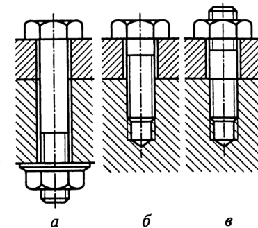
Рис. 1.6. Резьбовые соединения
