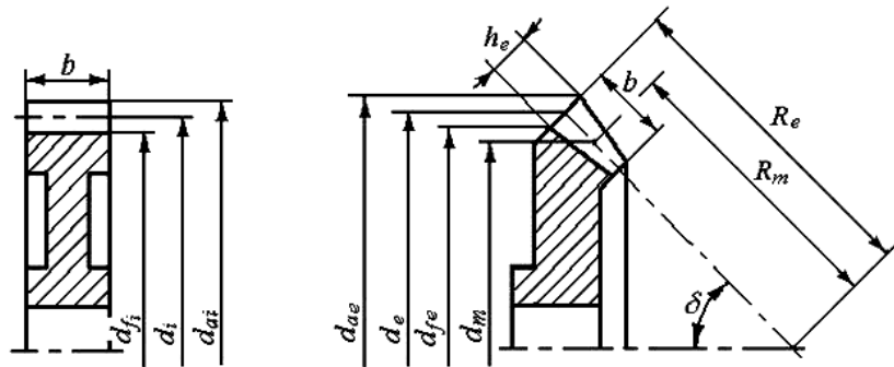
Рис. 6. Цилиндрическое колесо
