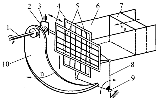
Рис. 3.4. Принципиальная схема режущего узла шпигорезки:
