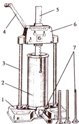
Рис. 4.6. Ручной шприц:
