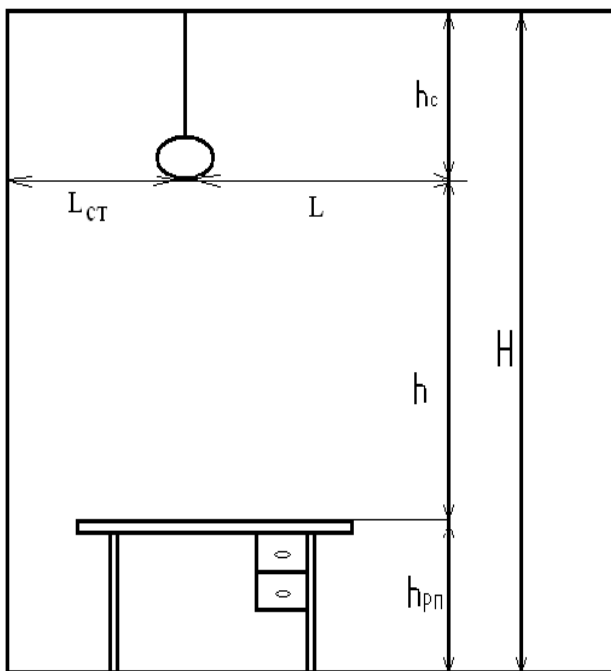
Рис. 2.2.5.1.1 Размещение светильников в помещении
