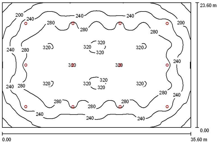
Рис. 2.2.5.4.2. Плоскостное распределение освещённости участка технического обслуживания
