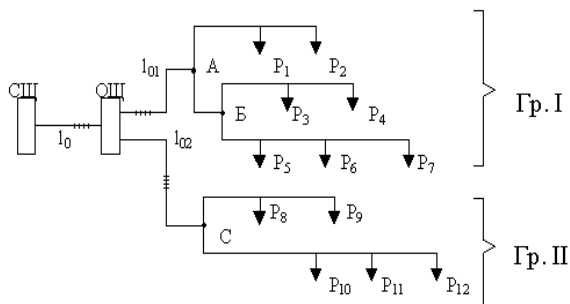
Рис. 2.3.2.1. Расчетная схема осветительной сети
