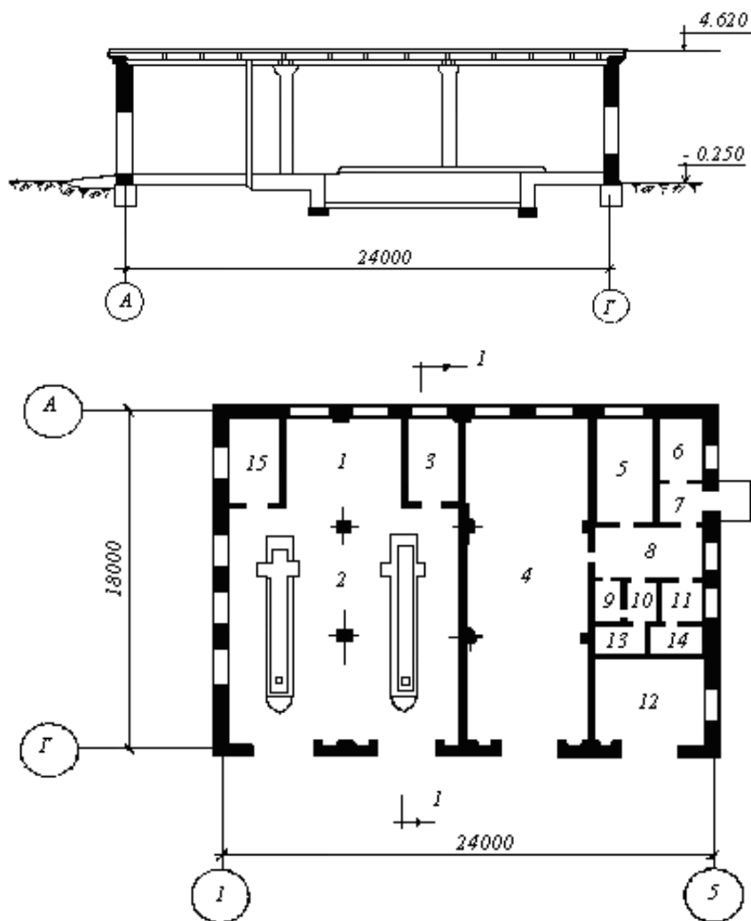
Объект-9. Секционное хранилище семенного картофеля емкостью 1000 т с активной вентиляцией
