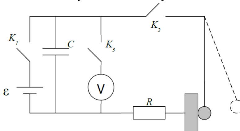
Рис.3. Электрическая схема установки
