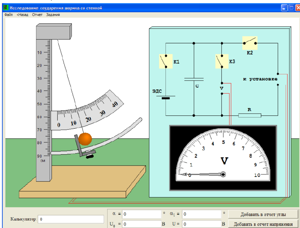
Рис.1. Основное окно программы и схема экспериментальной установки
