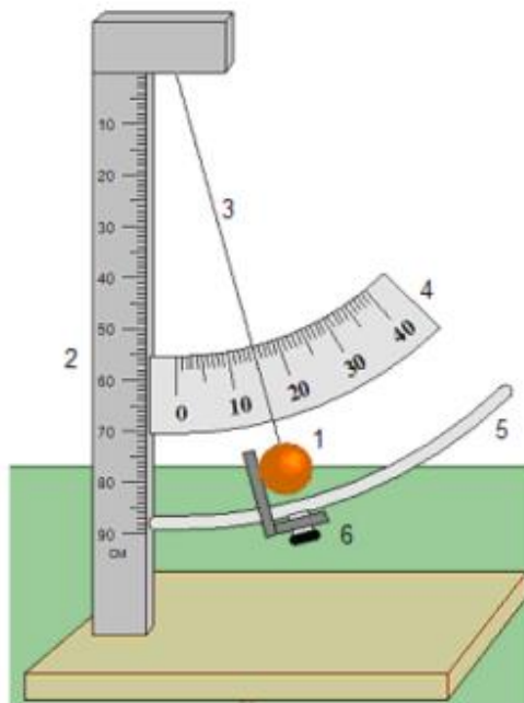
Рис.2. Механическая часть установки
