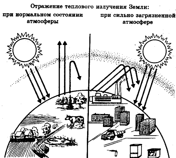
Рис. 3 Отражение теплового излучения Земли
