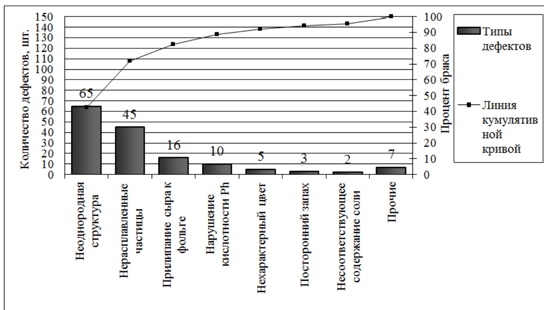
Рис. 1. Диаграмма Парето
