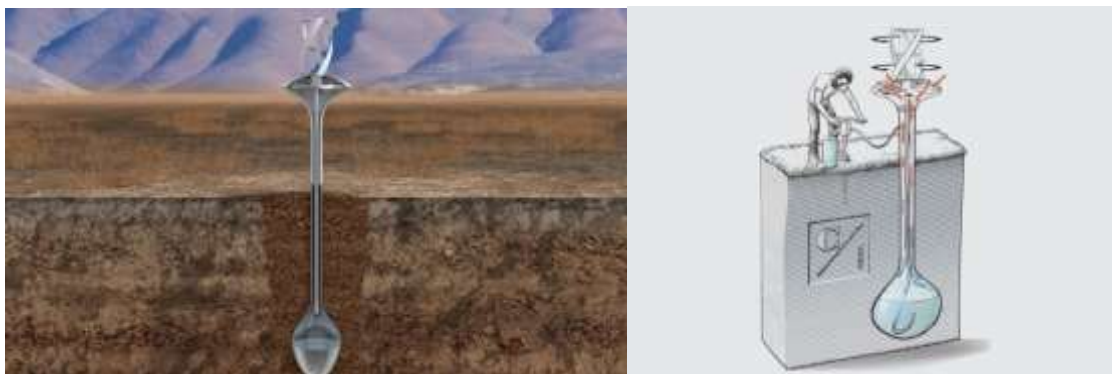
Рис. 2. Установка WaterSeer
