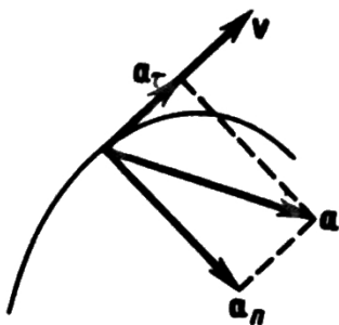
Рисунок 1.4. – Вектор ускорения
