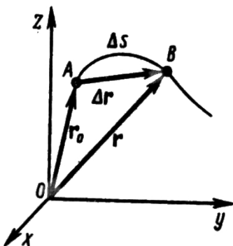
Рисунок 1.3. – Вектор перемещения
