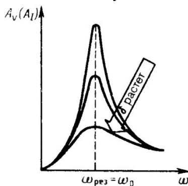
Рисунок 5.13. – Вынужденное колебание
