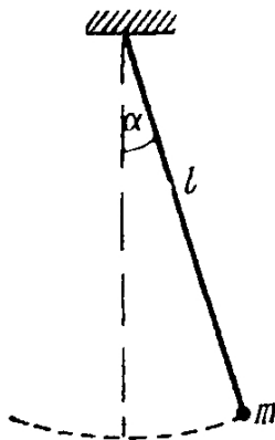
Рисунок 5.6. – Колебание груза
