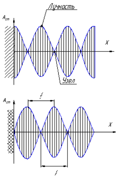
Рисунок 5.16. – Стоячие волны
