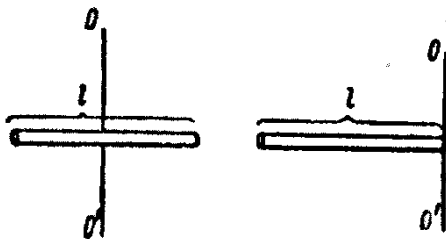
Рисунок 3.3. – Момент инерции стержня относительно оси, перпендикулярной стержню, проходящей через его середину и конец
