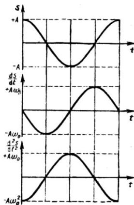
Рисунок 5.3. – Графики изменения кинематических характеристик ( y, v, a ) гармонического колебания со временем
