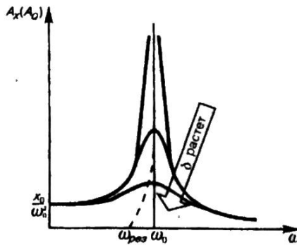
Рис.5.14. – Резонансные кривые
