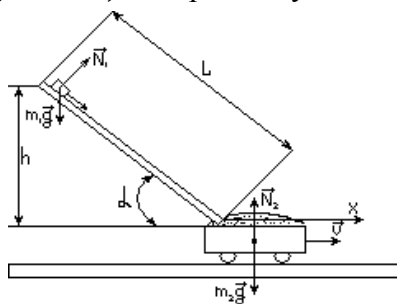
Рисунок 2.5. – Силы, действующие на тележку и ящик
