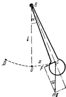
Рисунок 5.4. – Физический маятник
