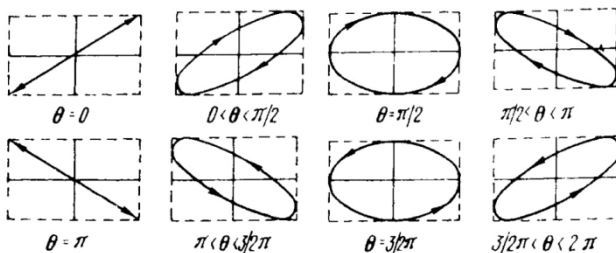
Рисунок 5.11. – Фигуры Лиссажу
