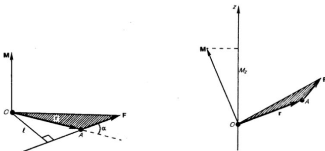
Рисунок 3.1. – Направление момента силы
