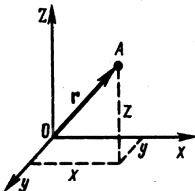
Рисунок 1.2. – Радиус-вектор
