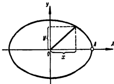
Рисунок 5.10. – Эллипс
