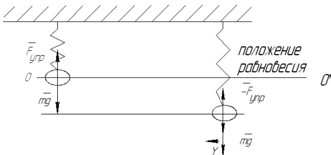
Рисунок 5.2. – Пружинный маятник
